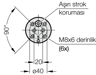
Görünüm X
