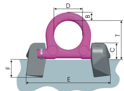
Abb. 6: Bemaßung
