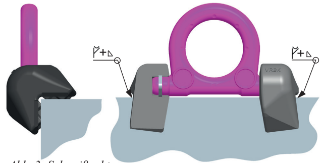
Abb. 3: Schweißnaht
